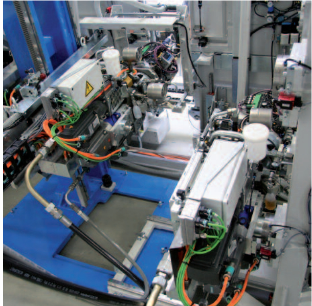
可选择的快速转换系统，保证自动转换材料无生产间断
