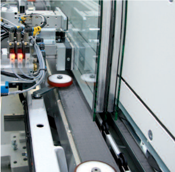
通过支撑滚轴自动调整，保护三层中空单元的中间玻璃
